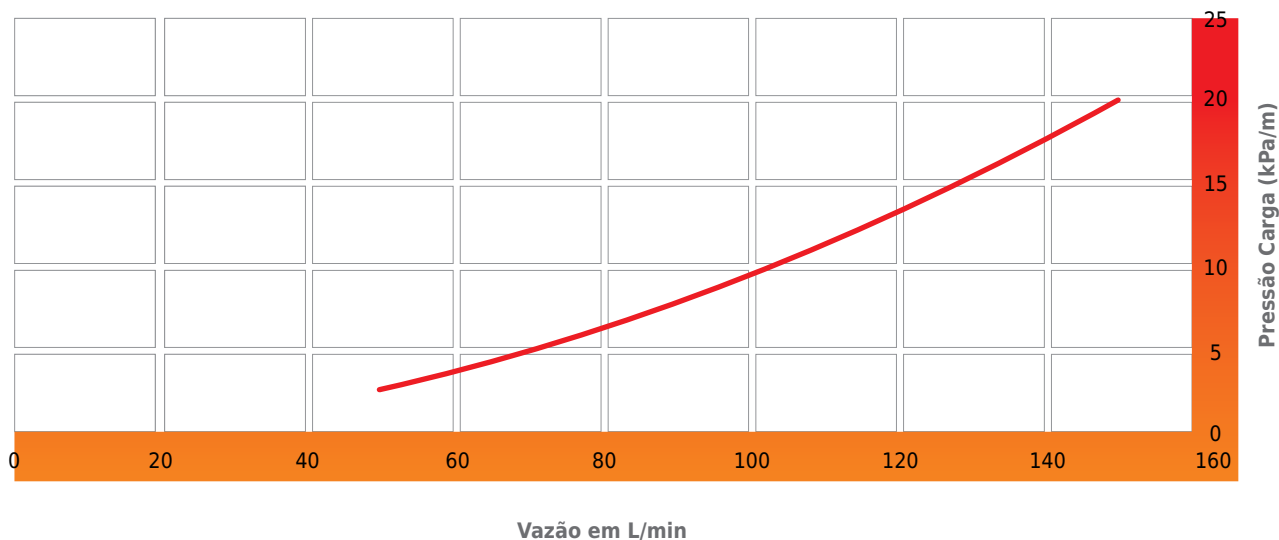
Perda de Carga da Mangueira Semirrígida
